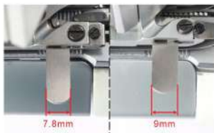
刀片宽度 Blade width
